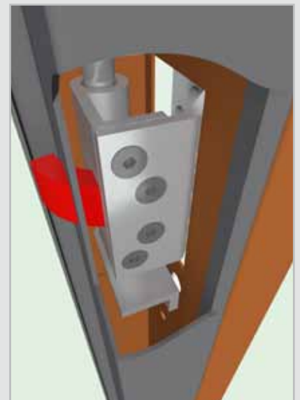
Particolare del rostro antistrappo che s'inserisce integralmente nel controtelaio.
